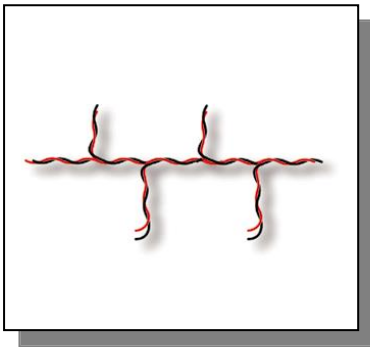
Durchgehend: Die beste Position für den SH2MCG24 wäre in der Mitte der Leitung.
