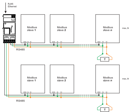
Fig. 1 Collegamento Modbus RTU Master COM 1, master COM 2
