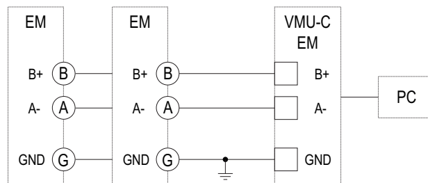
Fig. 2 RS485 COM2 vers compteur d'énergie
