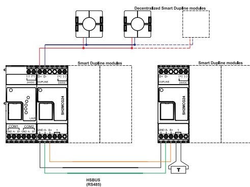
Fig. 3 Beispiel für Verbindung von Smart-Dupline-Modulen vermittels Master-Kanalgeneratoren
