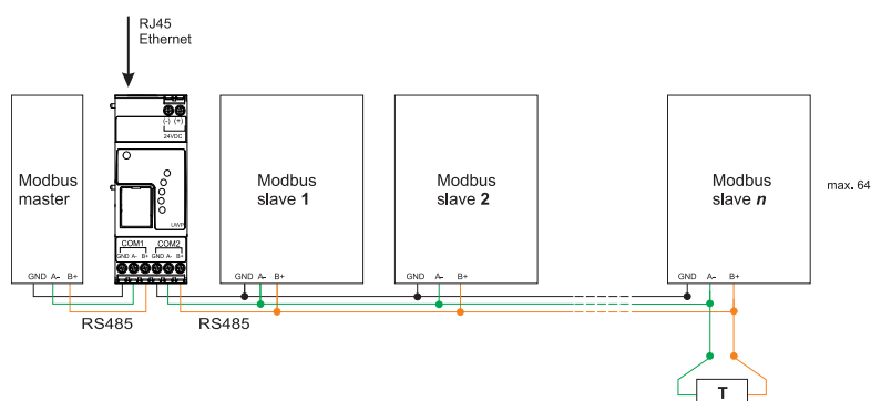
Fig. 2 Modbus RTU tilslutning. COM 1 slave, COM 2 slave
