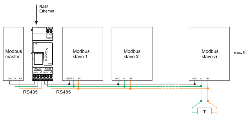
Fig.2 Modbus RTU 连接 COM 1 从、COM 2 主
