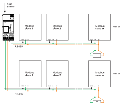
Fig.1 Modbus RTU 连接 COM 1 主、COM 2 主
